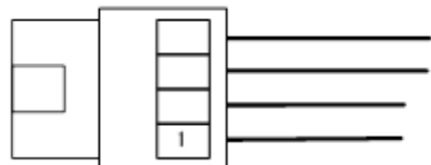
クイックコネクタ側の配線 (クイックコネクタを上方から見た図)
