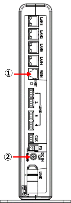
本装置 SG2000is4/is8 背面図
