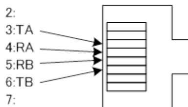
LANケーブル/RJ-45コネクタ側の配線 (RJ-45コネクタを先端から見た図)
